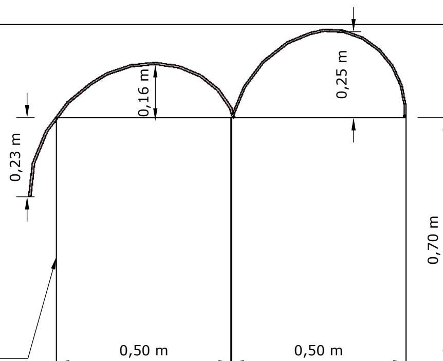
ELEVAÇÃO FRONTAL
